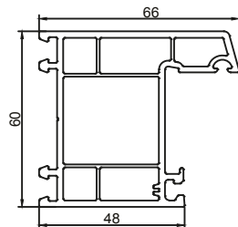
AP 202 CASEMENT DOOR OUTER FRAME
