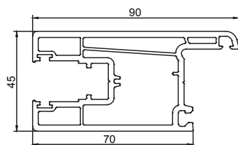
AP 305 SLIDING DOOR SASH
