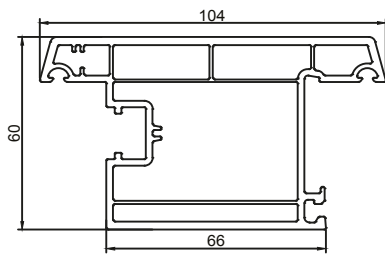
AP 205 CASEMENT DOOR SASH
