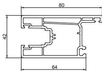
AP 105 SLIDING DOOR SASH
